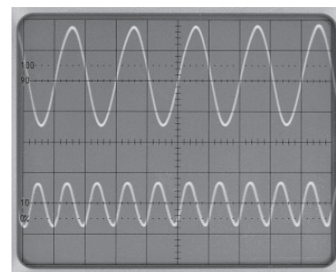
50MHz und 100MHz Sinus-Signal mit alternierender Triggerung
